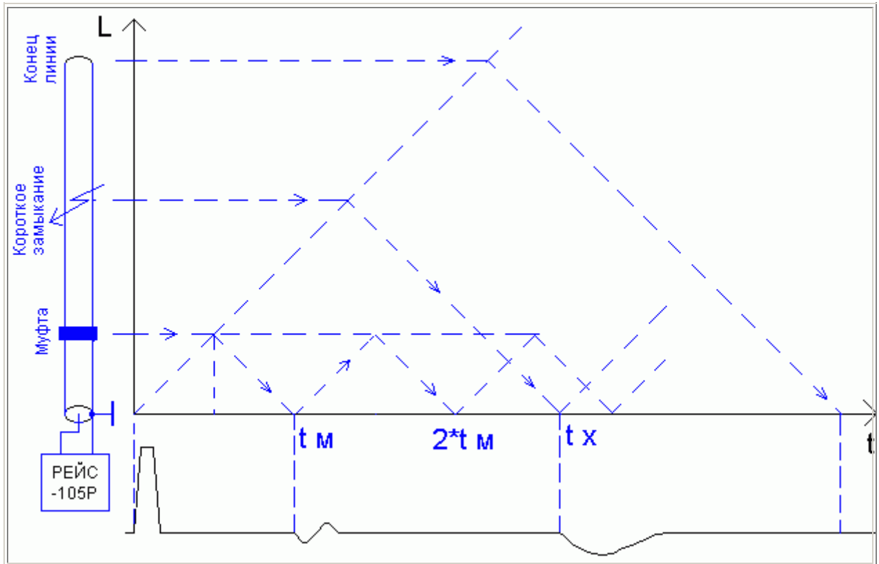
Рисунок 2 - Рефлектометрический метод определения места повреждения
